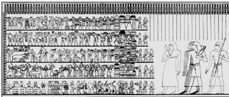
Рис. 2. Сцена принесення іноземцями дарів із гробниці Рехміра (Т. 100). Тутмос III-Аменхотеп II. XVIII династія [16]
